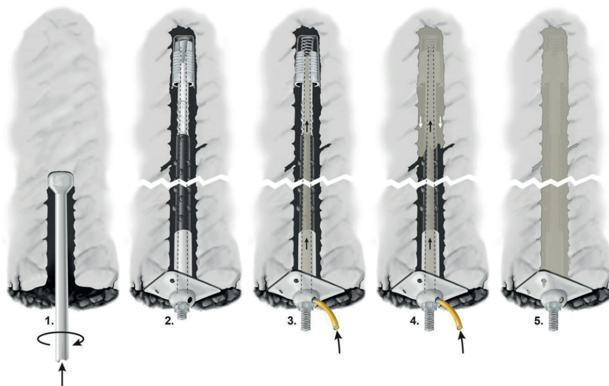
Figur 4.15 Montering av kombinasjonsbolt
