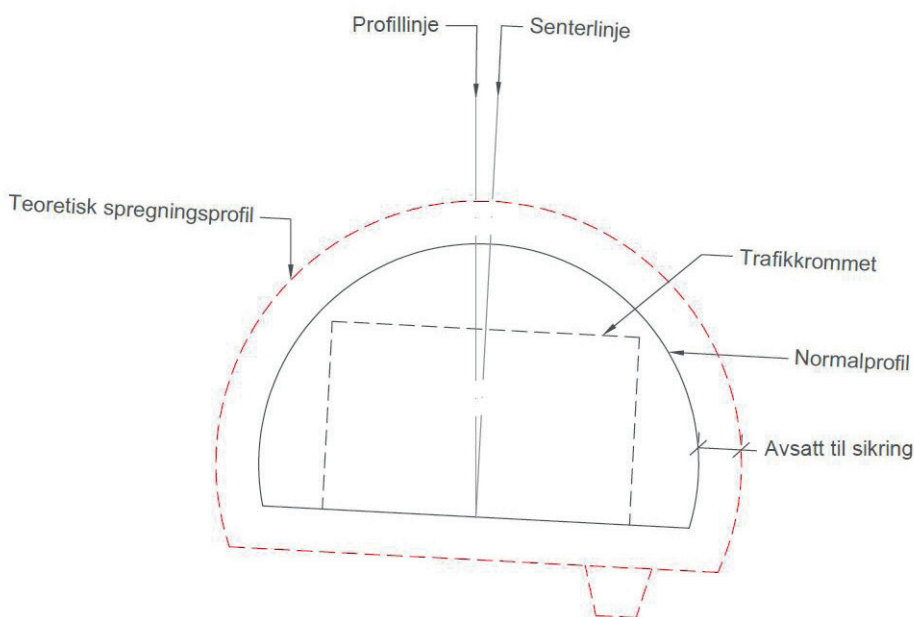
Figur 7.4 Sjematisk tunnelprofil, stiplet rød linje er teoretisk sprenningsprofil med sideveis helning.
