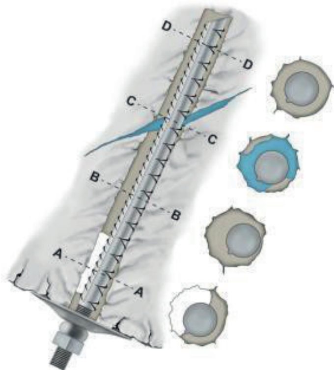
Figur 3.3 Eksempler på kvalitetsavvik på innstøpte bolter
