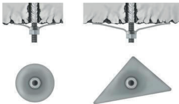
Figur 3.2 Eksempler på underlagsplater
