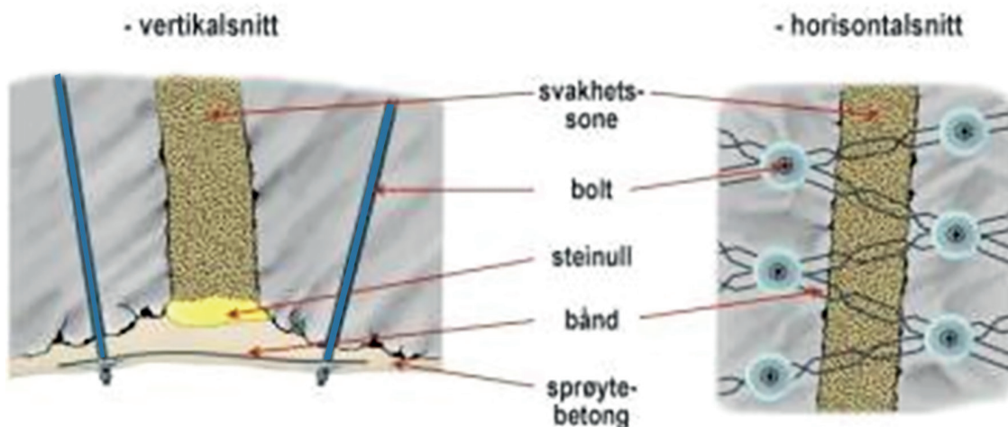
Figur 2.12 Eksempler på bolting i slepper og svakhetssoner
