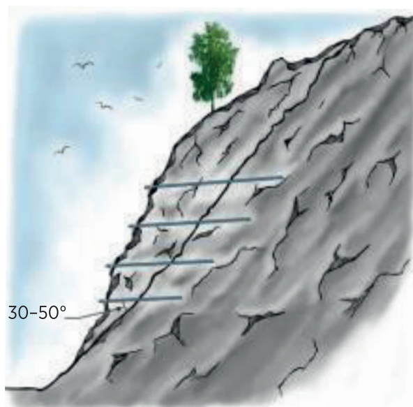
Figur 5.10 Anbefalt vinkel mellom bolt og sprekkeplan
