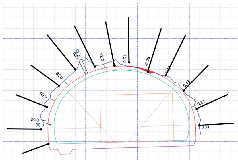
Figur 7.12. Teoretisk sprengningskontur (grønn) mot faktisk sprengningskontur (rød). Knølen er vist som rødt område /29/.
