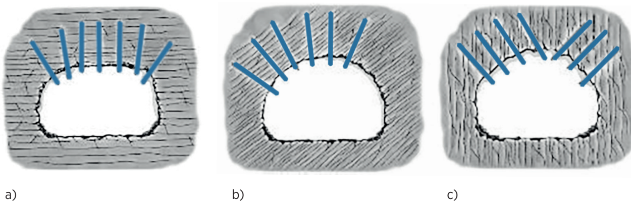
Figur 2.9 Eksempler på bolting i lagdelt/skifrig berg, a) horisontalt, b) skråtilt og c) vertikalt
