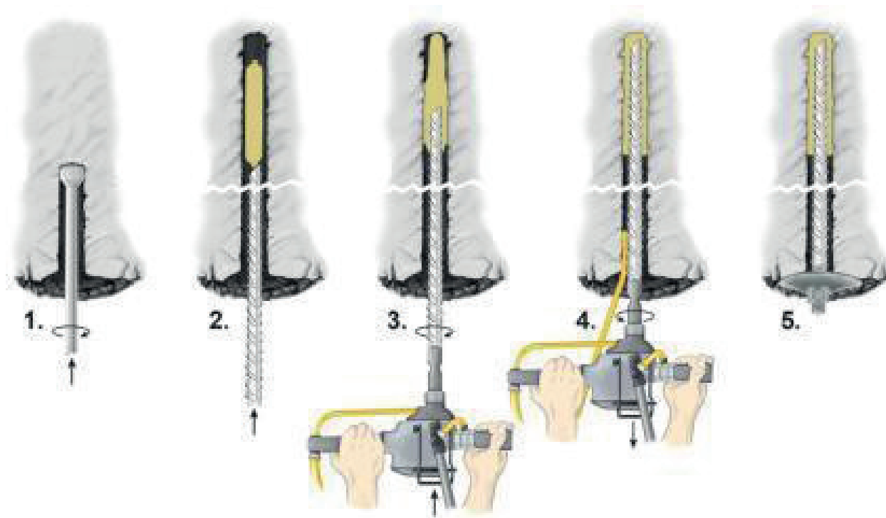
Figur 4.10 Montering av bolt med polyesterpatron (endeforankrede bolter)
